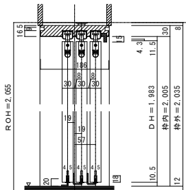
■縦断面図
