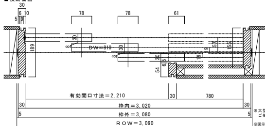
■横断面図
