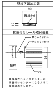
■縦断面図[床直付けレールタイプ]
