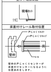
■調整枠下加工図
