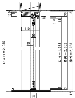
■調整枠下加工図
