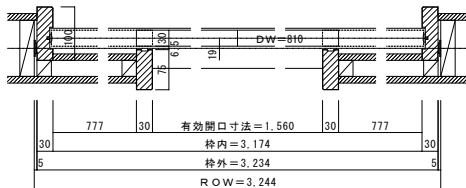
■横断面図
