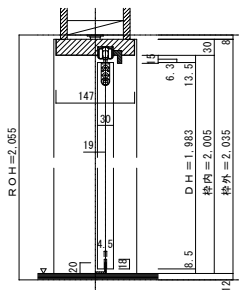
■縦断面図
