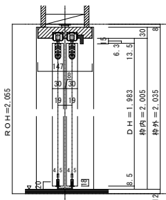
■縦断面図
