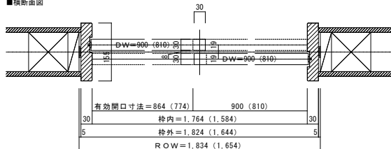
■横断面図
