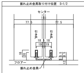
振れ止め金具取り付け位置 S=1/2
