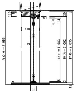
■縦断面図[床直付けレールタイプ]
