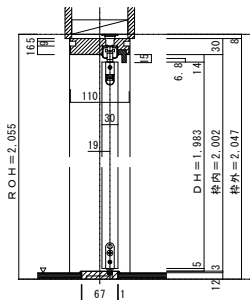
■縦断面図[レールタイプ]
