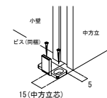
振れ止め金具(床付け用)取り付け
