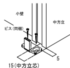
振れ止め金具(床付け用)取り付け
