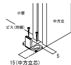
振れ止め金具(床付け用)取り付け
