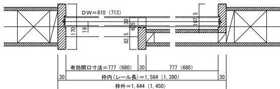
■横断面図
