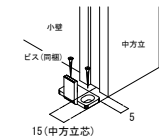
振れ止め金具(床付け用)取り付け
