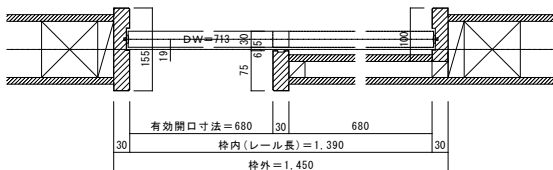
■横断面図
