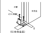
振れ止め金具(床付け用)取り付け
