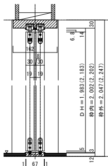
■縦断面図[L-タイプ]
