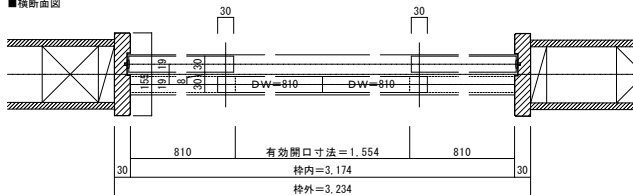
■横断面図
