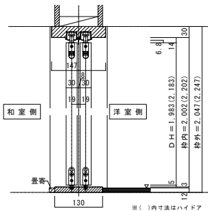
■縦断面図[レールタイプ]
