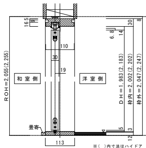
■縦断面図[L-タイプ]
