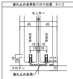
振れ止め金具取り付け位置 S=1/2
