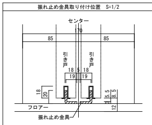
揺れ止め金具取り付け位置 S=1/2
