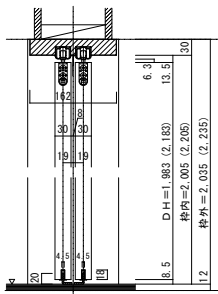
■縦断面図
