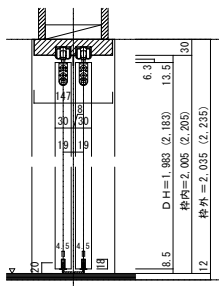
■縦断面図
