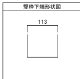
壁枠下端形状図
