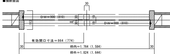
■横断面図
