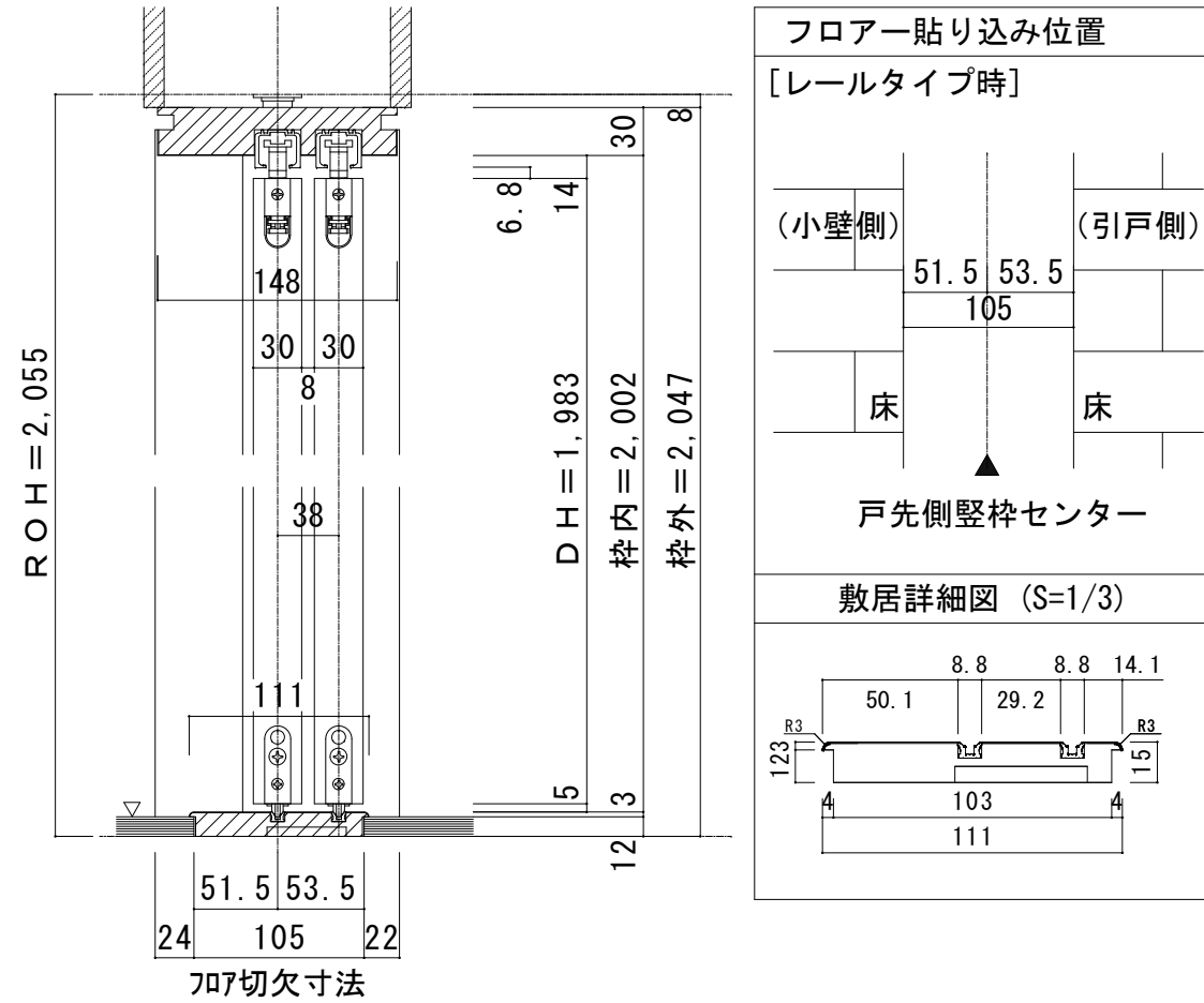
B-B断面図
