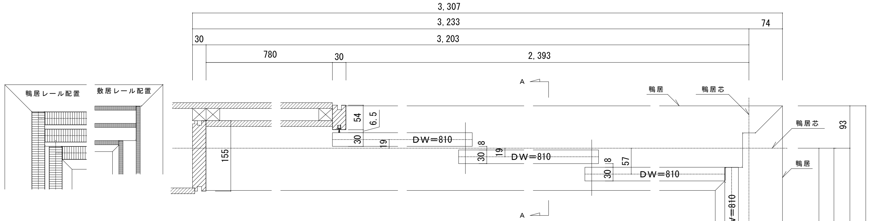
B-B断面図
