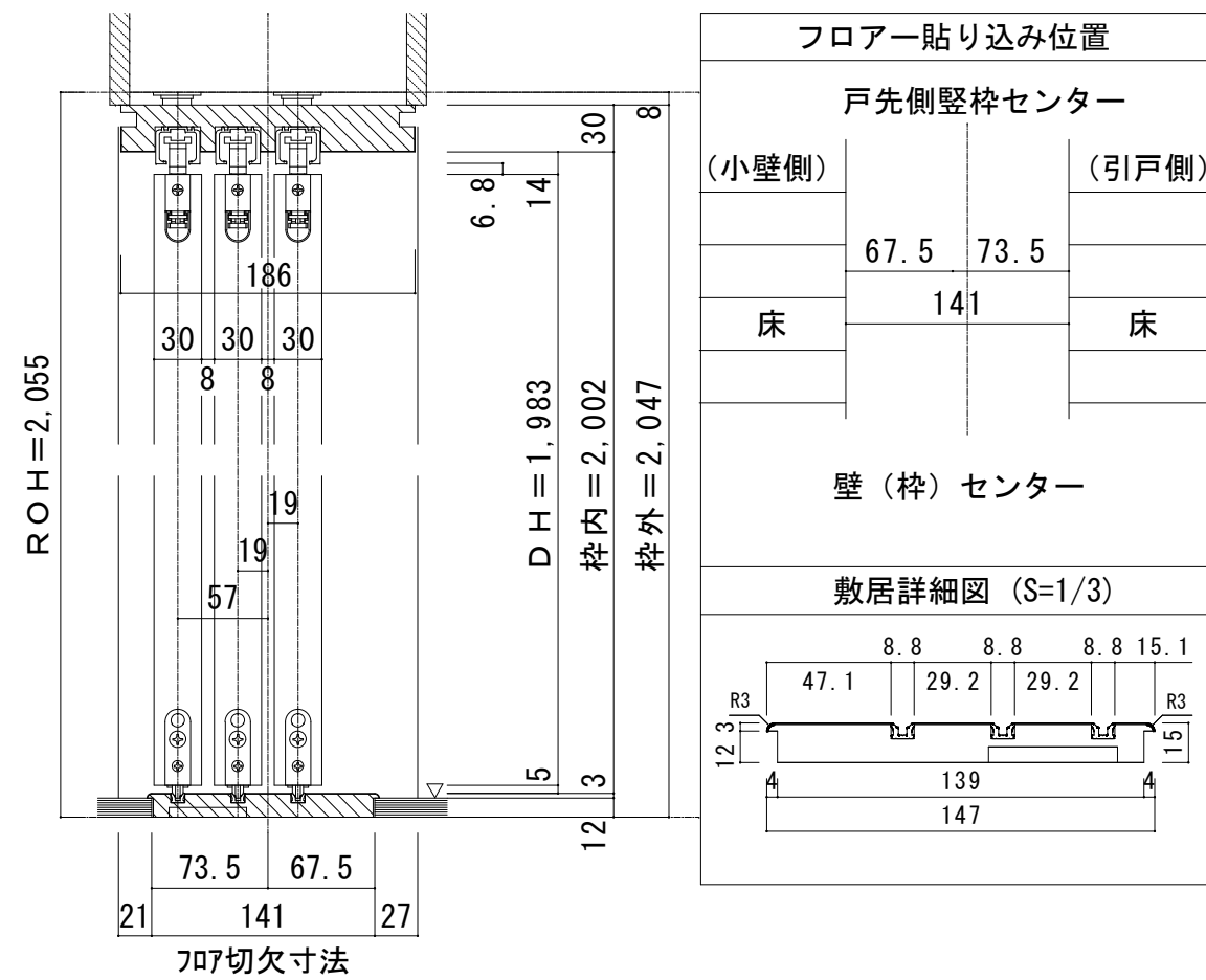
A-A断面図
