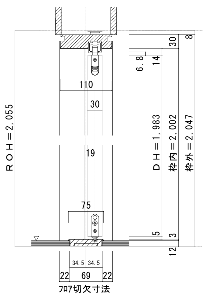
B-B断面図
