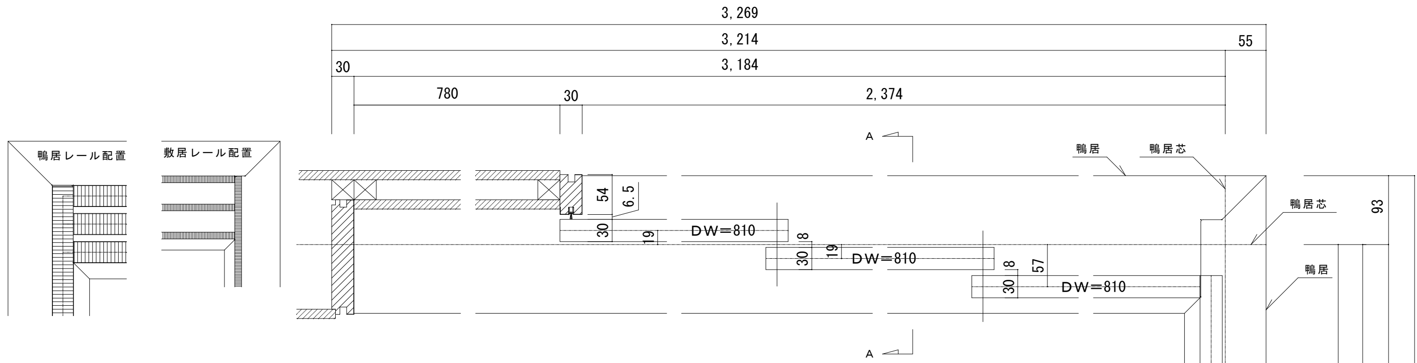
A-A断面図
