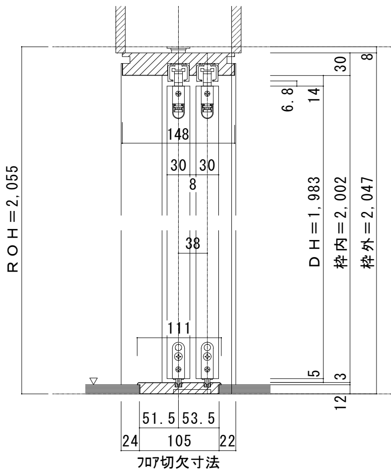
A-A断面図
