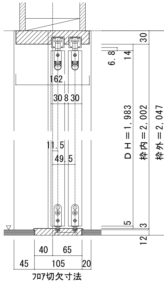
B-B断面図
