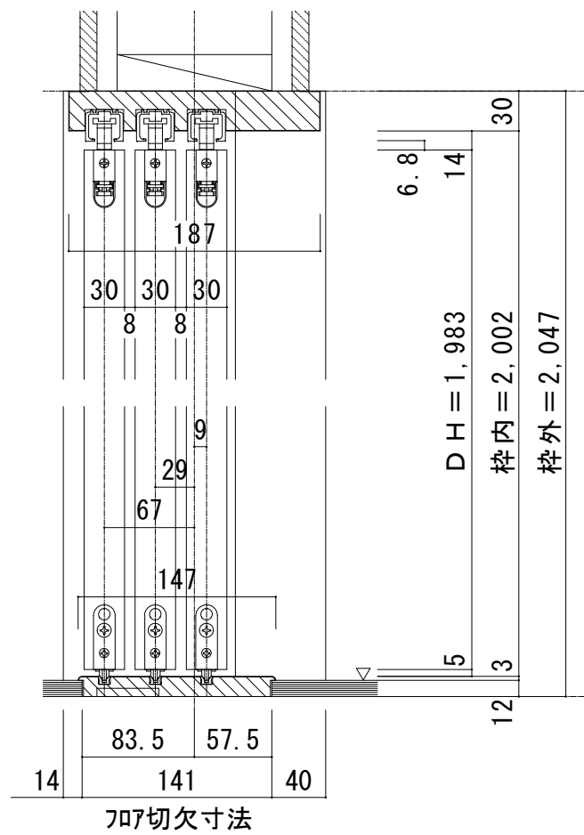
A-A断面図
