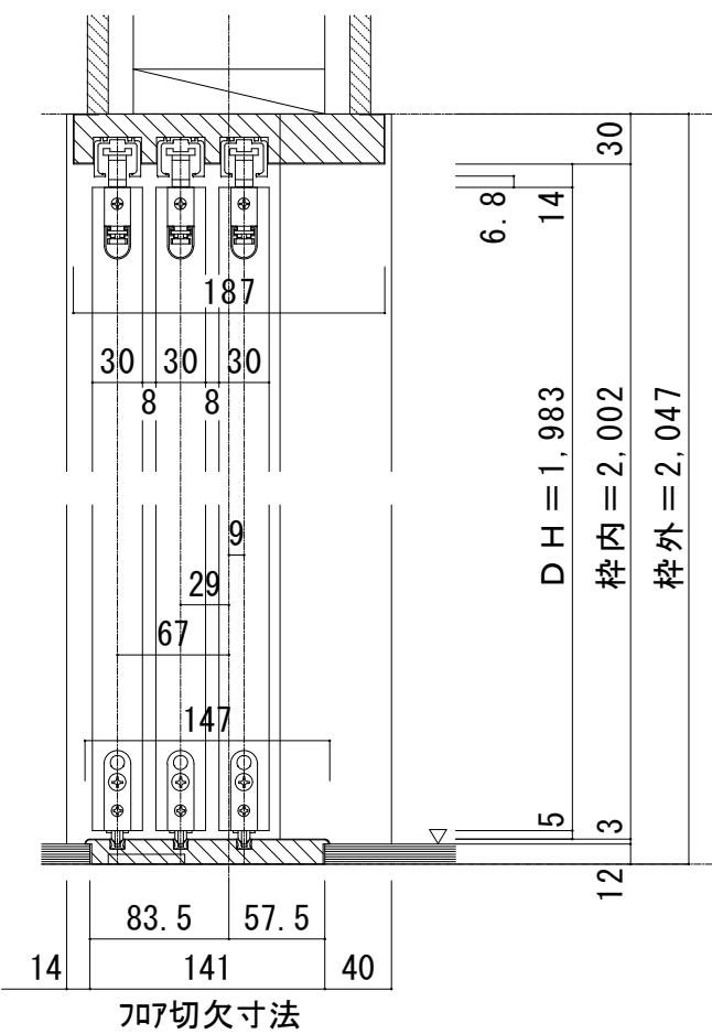
A-A断面図
