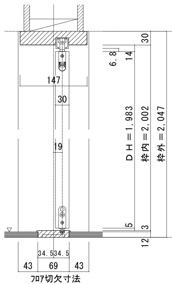
B-B断面図
