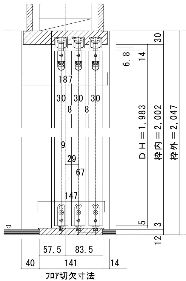
A-A断面図
