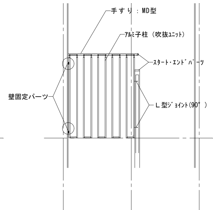
吹抜 立面図
