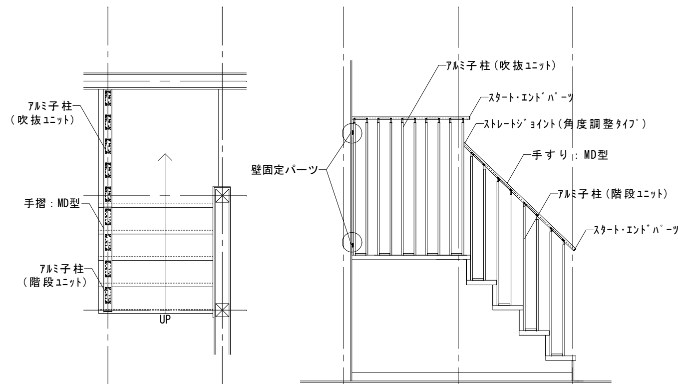
平面図
