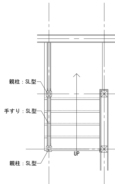
平面図
