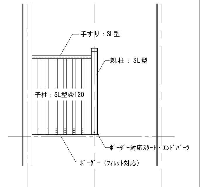
吹抜け面 手摺詳細図
