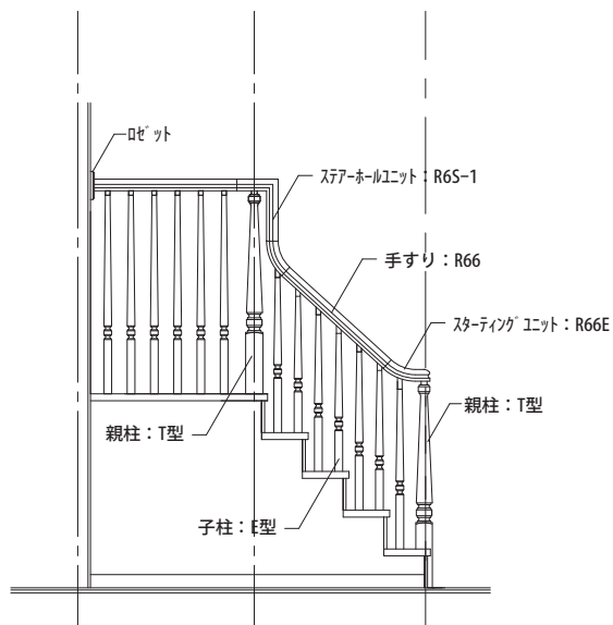
立面図
