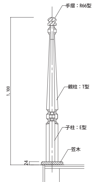
吹抜け面 手摺詳細図
