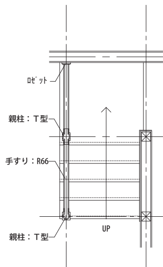
平面図
