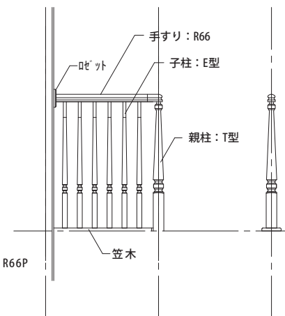
吹抜け面 手摺詳細図
