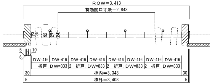
■横断面図
