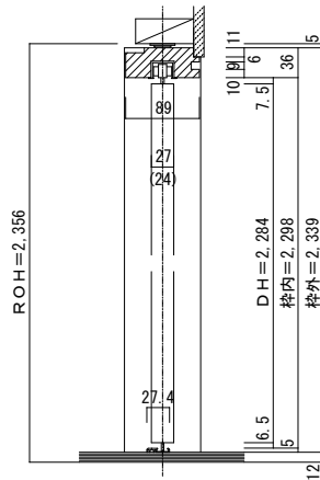
■縦断面図 [3方枠+床直付レール]
