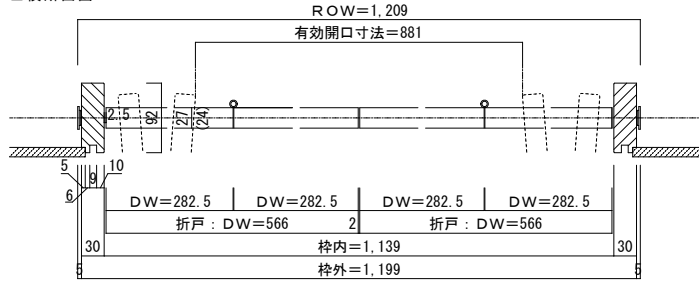
■横断面図
