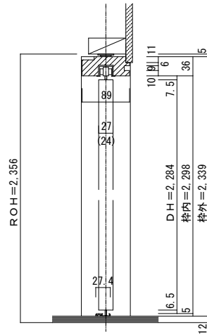
■縦断面図
