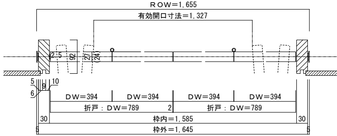
■横断面図
