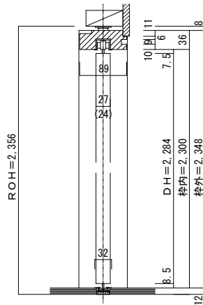
■縦断面図
