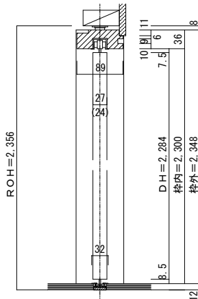
■縦断面図
