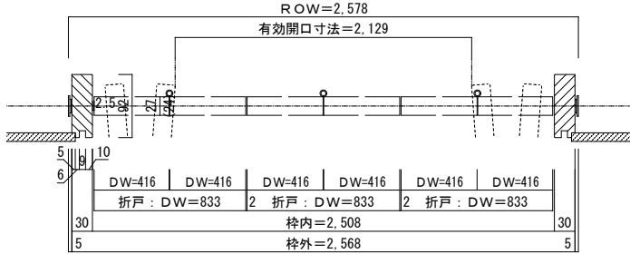
■横断面図
