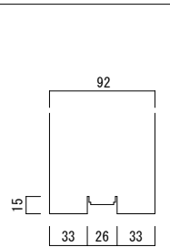
■ 縦枠下端形状図 (S=1/3)
