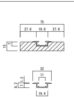
■ 下枠詳細図 (S=1/2)
