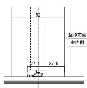
■ 床直付レール取り付け位置 (S=1/2)
