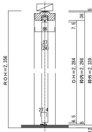
■縦断面図
