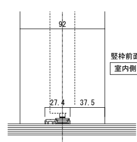
■ 床直付レール取り付け位置 (S=1/2)
