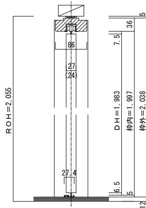
■縦断面図
