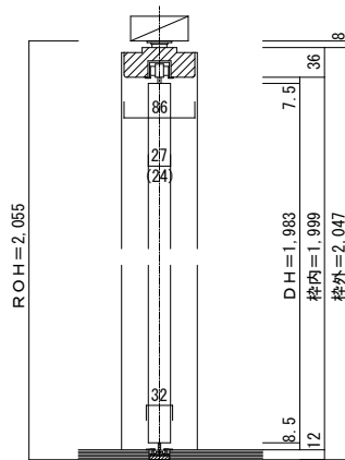
■縦断面図
