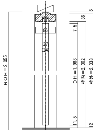
■縦断面図 [3方枠]
