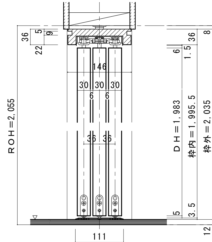
■縦断面図 [床直付けレールタイプ]
