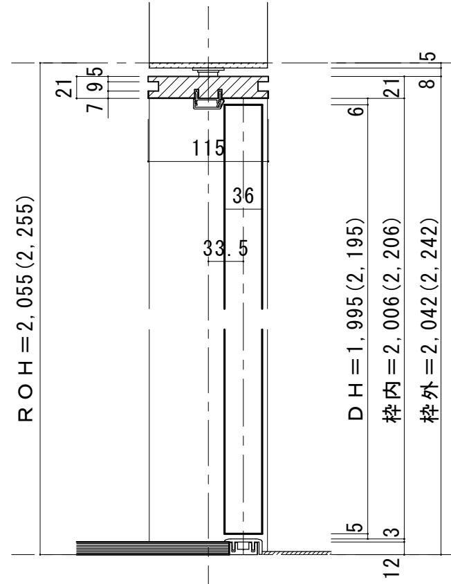
■ 縦断面図 [片ツハタイプ]
