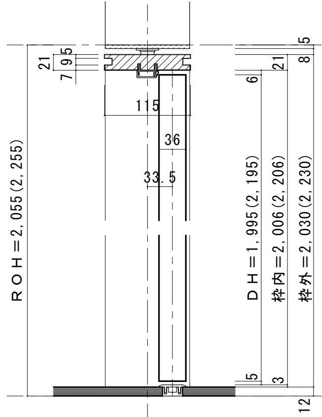
■ 縦断面図 [両ツハタイプ]
