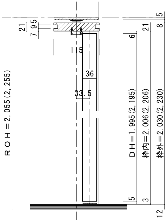
■縦断面図
