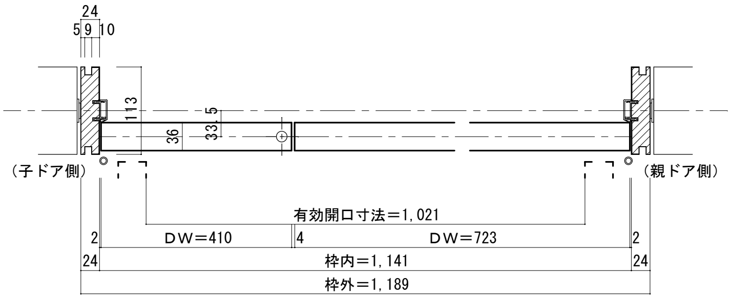
■横断面図
