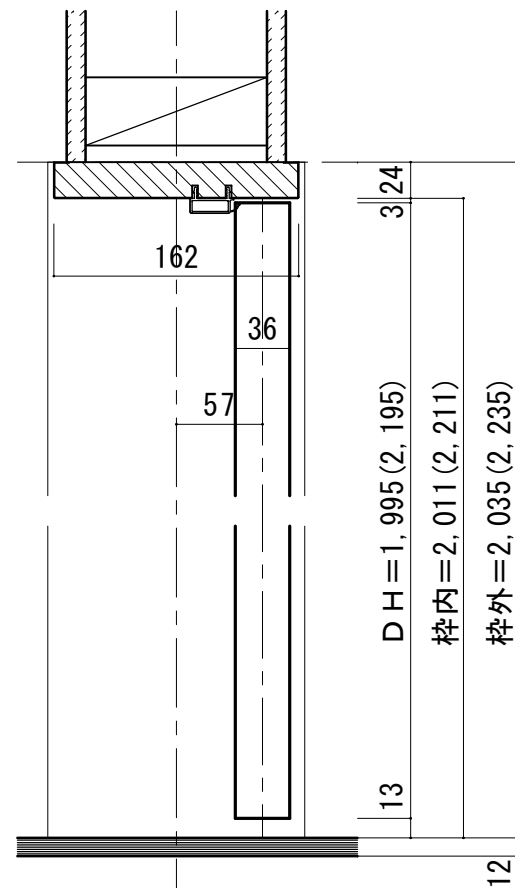
■縦断面図
