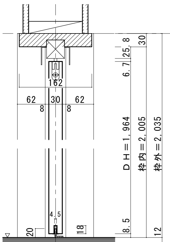
■縦断面図
