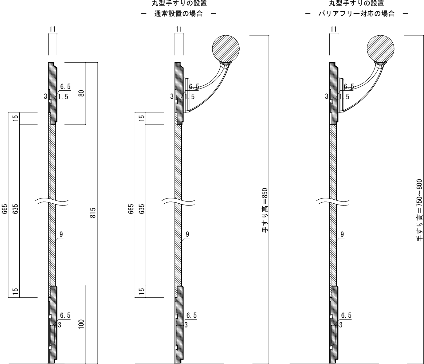
ストライプパネル縦断面図
