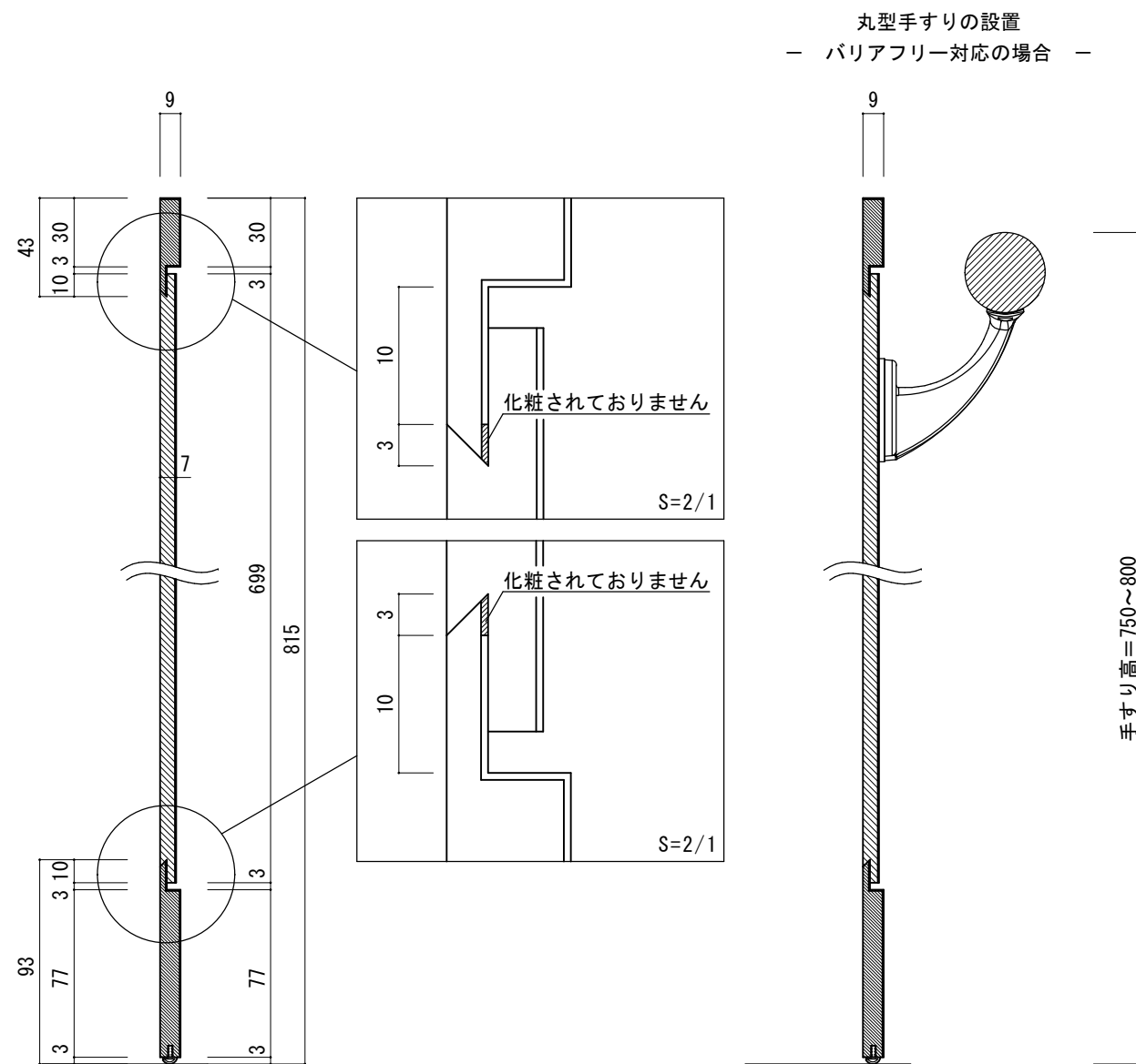
シンプルモダンパネル縦断面図
