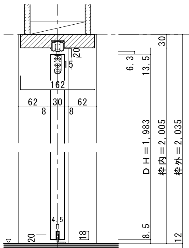
■縦断面図
